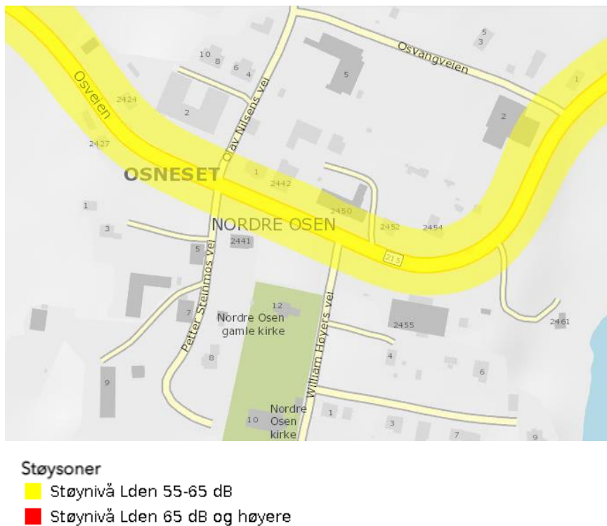
Figur 4-10. Støyvarselkart veg. Kilde: Støysoner for riks og fylkesveger – Statens vegvesen
